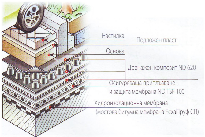
СИСТЕМА ПАРКИНГ - ПОКРИВ ЗА ЛЕКИ КОЛИ
