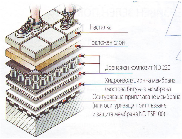
СИСТЕМА ПЕШЕХОДНА ЗОНА (СПАБО НАТОВАРЕНА)
