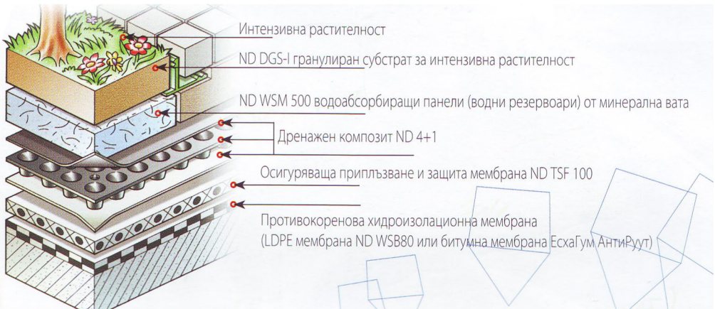
СИСТЕМА ИНТЕНЗИВЕН ЗЕЛЕН ПОКРИВ
